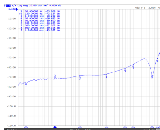
PSRR @30mA
