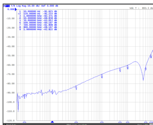
PSRR @30mA
