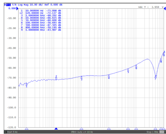
PSRR @30mA
