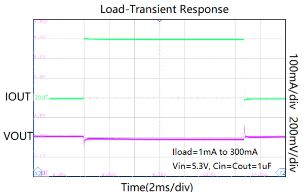
负载瞬态
