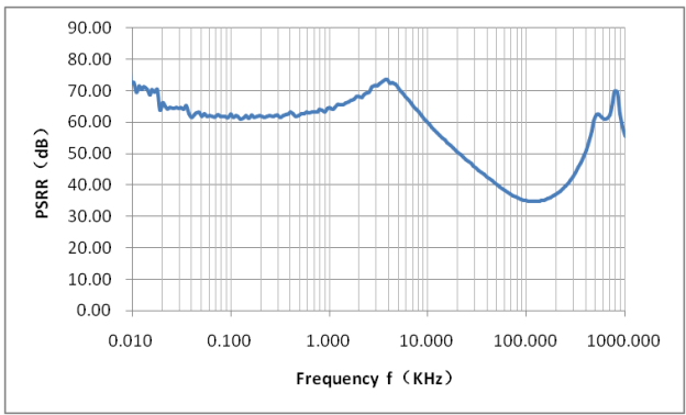
电源纹波抑制与频率间的关系
