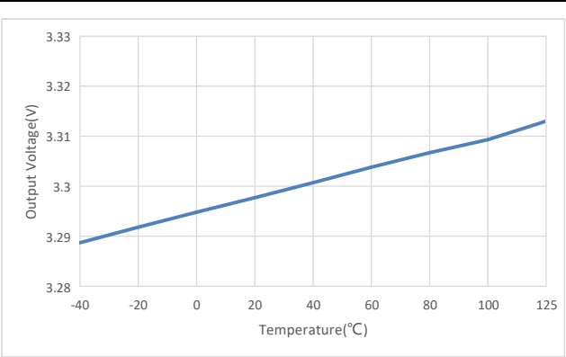
输出电压与温度间的关系, 其中 I_{OUT}=1mA
