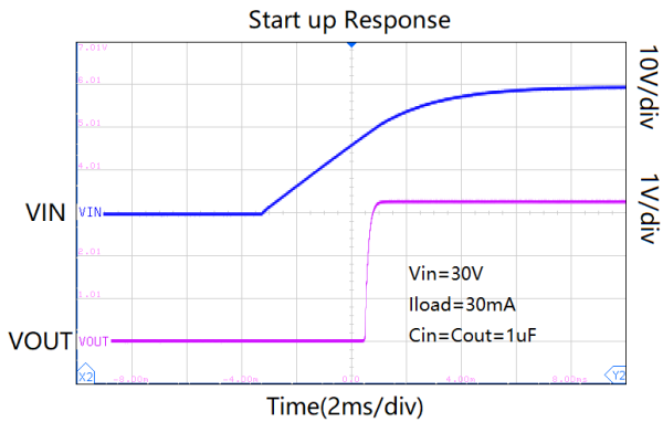
启动波形
