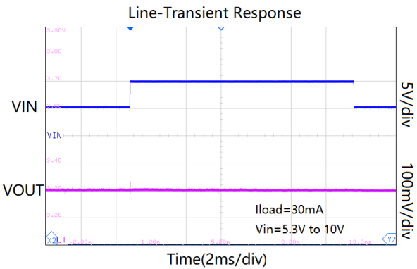
电源瞬态
